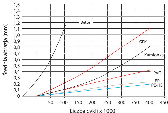
Średnia abrazja (zużycie ściernie) dla różnych materiałów. Wykres ścieralności met. Darmstadt
