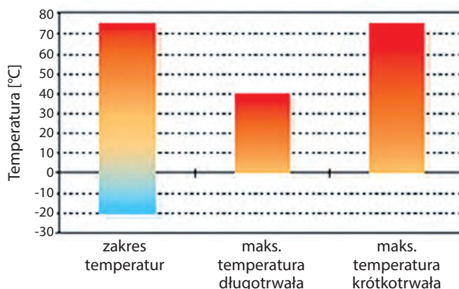
Zakres dopuszczalnych temperatur dla rur PE-HD
